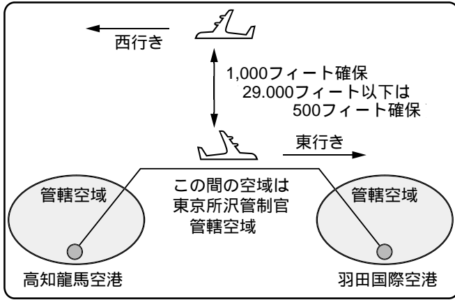
高度による安全確保・無線交信管轄略図
