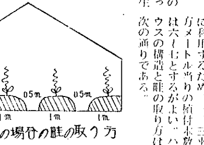
床中5.5mの場合の取のり方
