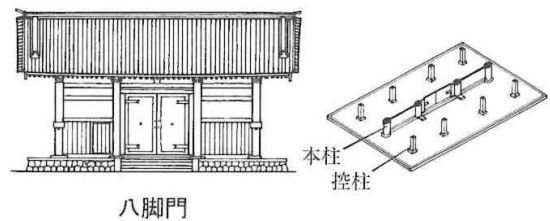
門の構造
