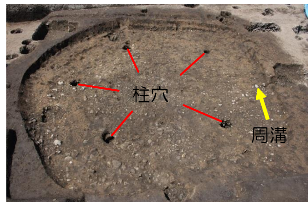
竪穴建物跡 完掘状況
