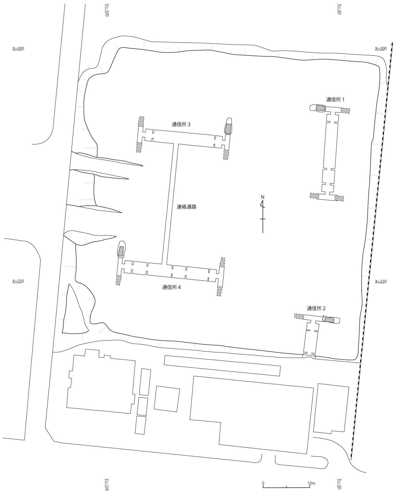
通信所跡 配置図
