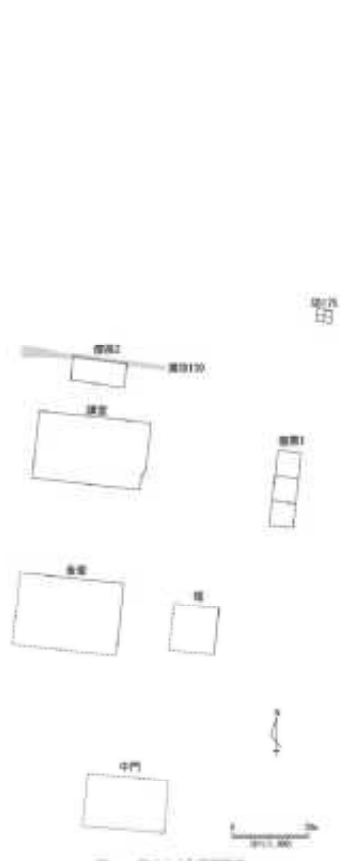
图3 野中廃寺伽藍配置図
