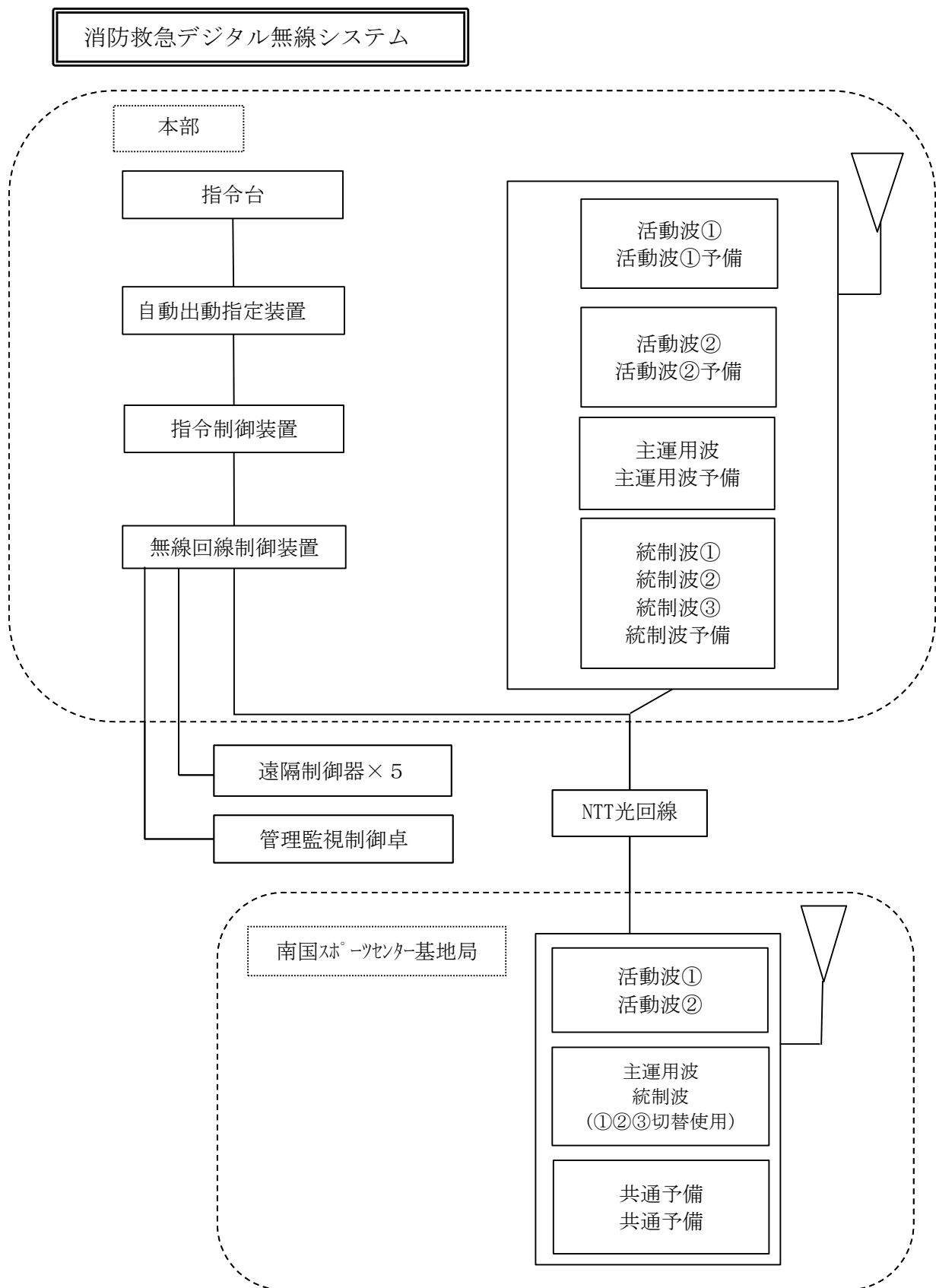
消防通信系統図(3)
