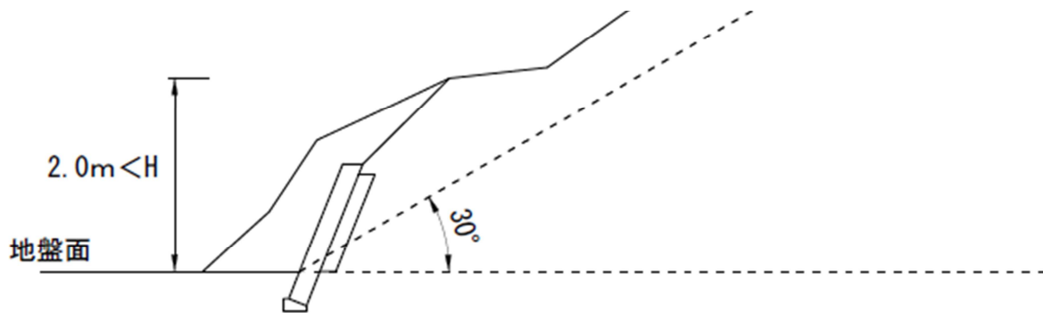
(ア) 切土をした土地の部分に生ずる高さが 2 m を超えるがけのがけ面
