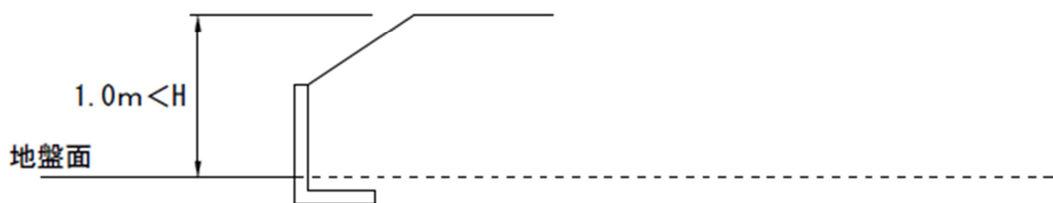
(イ) 盛土とした土地の部分に生ずる高さが 1 m を超えるがけのがけ面
