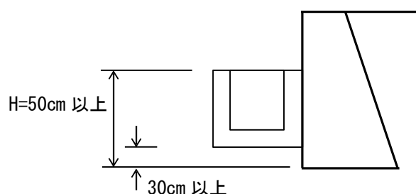
(c) 施設に隣接して設置する場合
