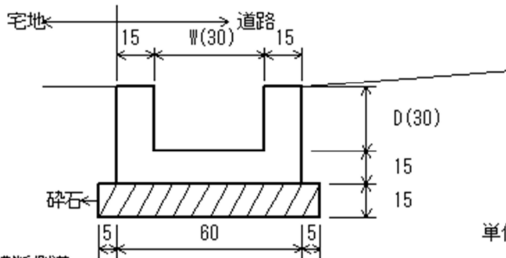
b 横断側溝
