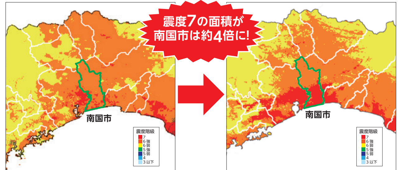
震度分布図(最大クラス重ね合わせ) 左:平成24年12月 右:令和7年10月
