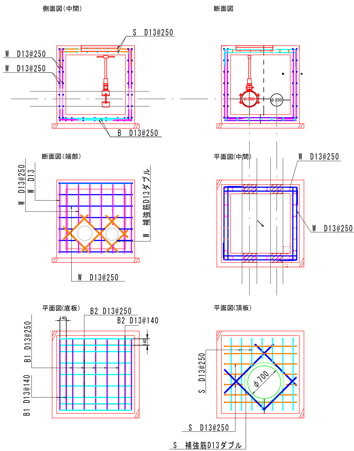
流量計室構造図 S=1:50
