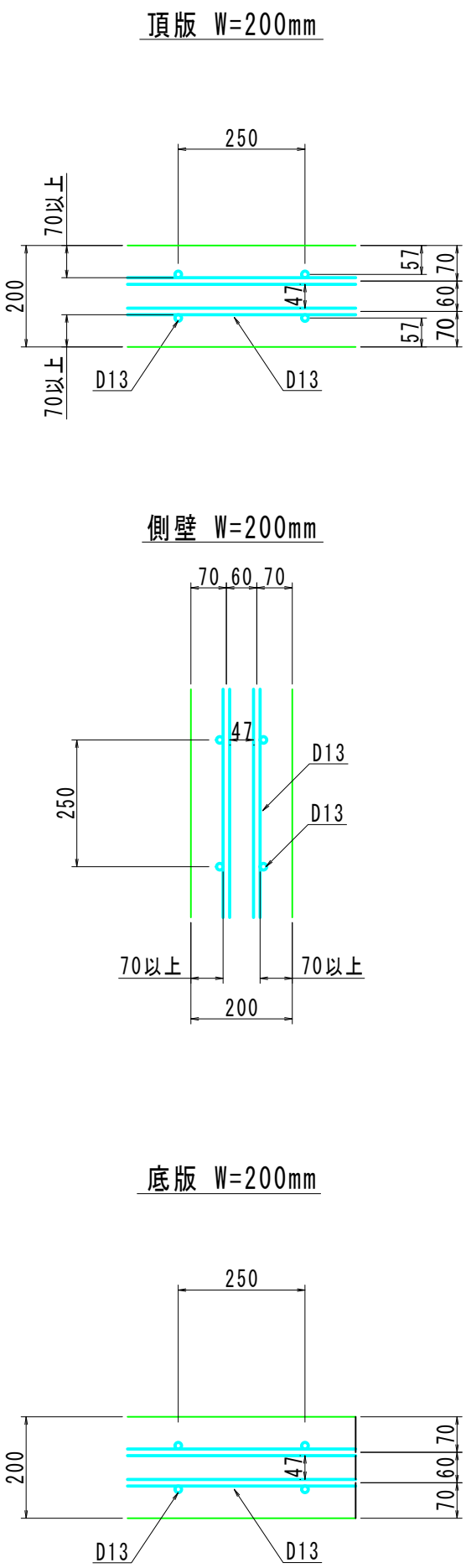
配筋かぶり標準図
