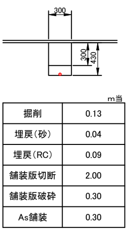
ケーブル埋設工 L=30.0m
