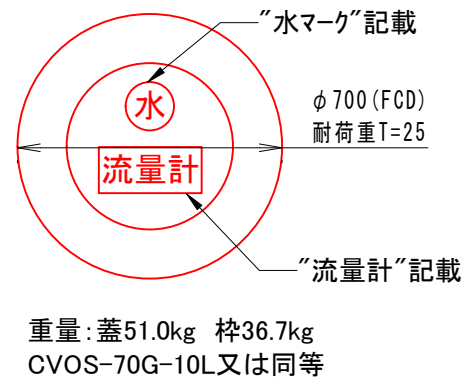
鉄蓋詳細図
