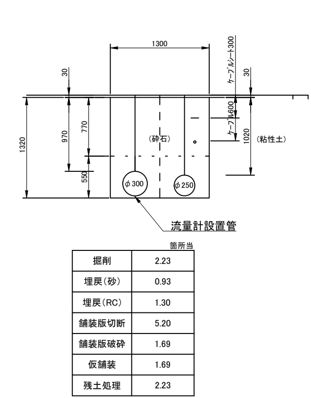
既設管断面図・試掘工 L=1.30m
