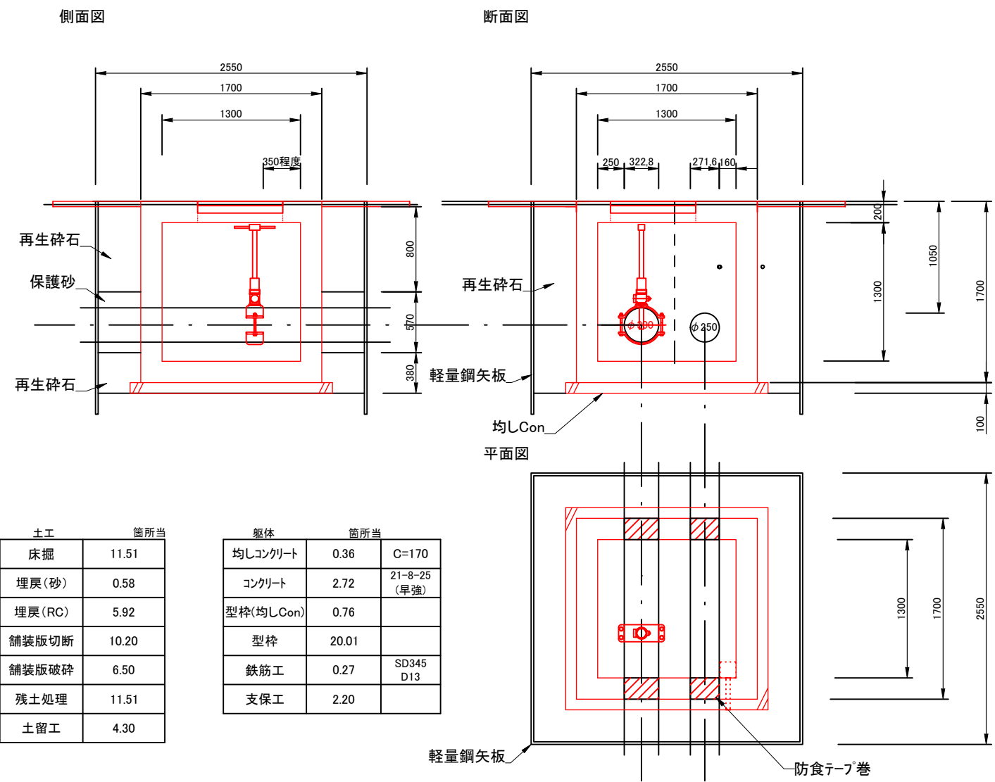
流量計室断面図 S=1:50
