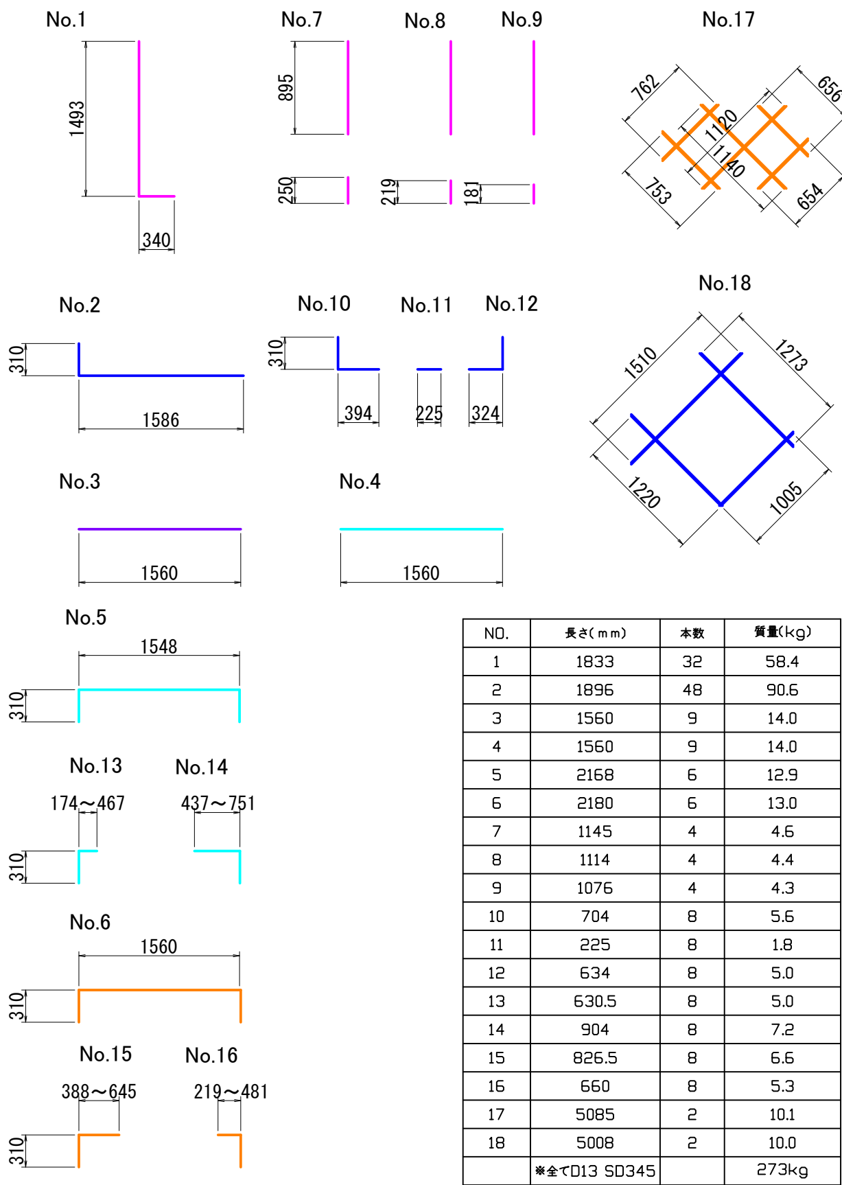
鉄筋詳細図
