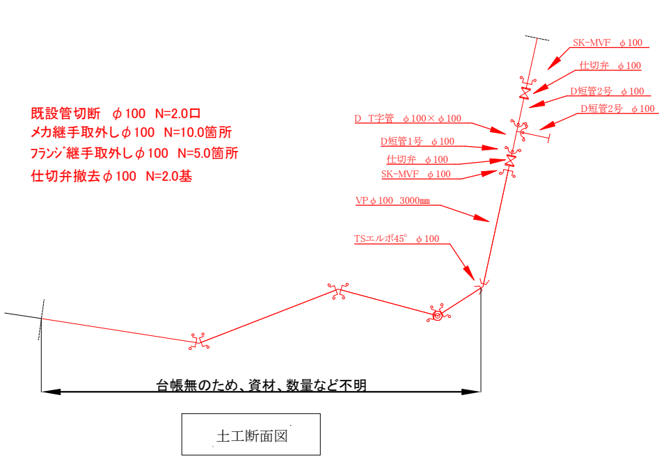
既設管撤去図
