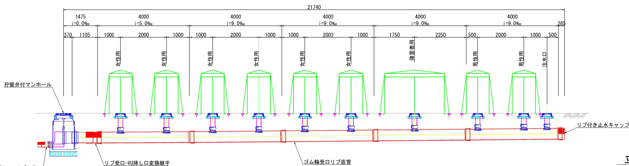
縦断図
