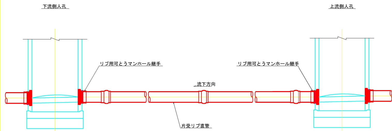
管布設工標準断面図
