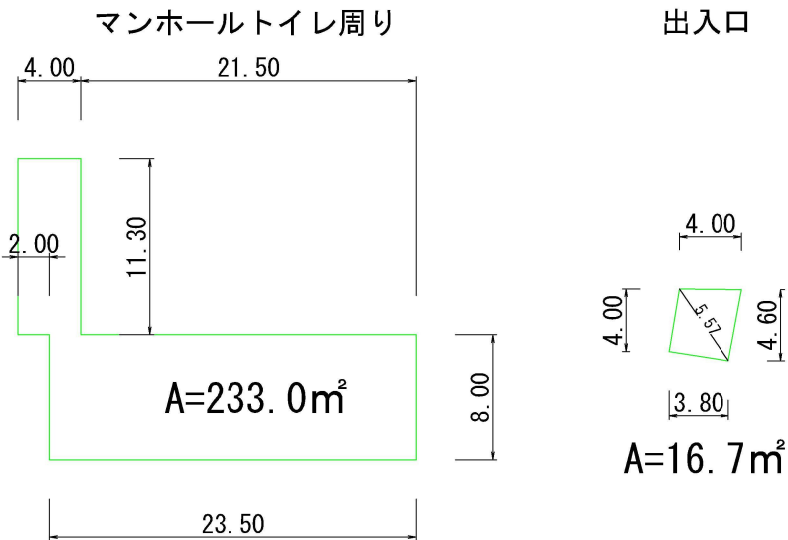
As舗装展開図 S=1:500
