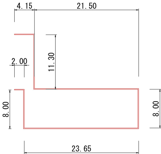
地先境界ブロック平面図 S=1:500 L=78.6m
