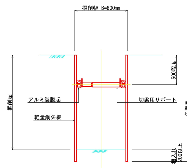
支保工 1 段
