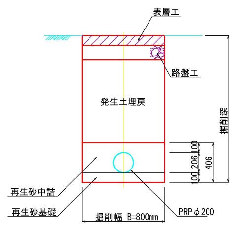
土工定規断面図
