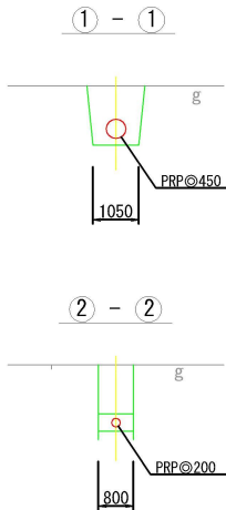
横断面図 S=1:200
