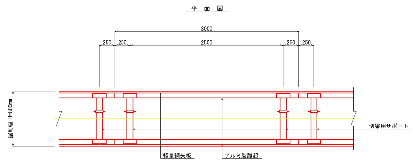
支保工 1 段
