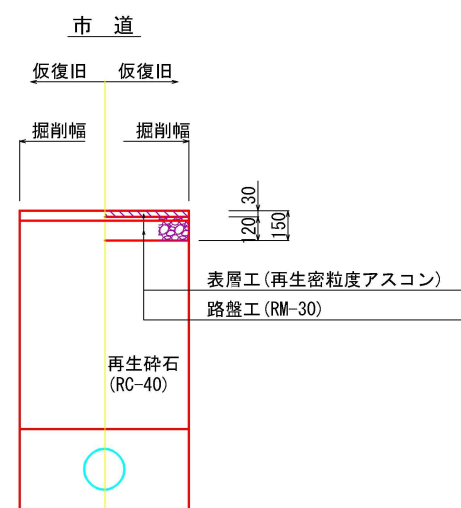
路面復旧標準図
