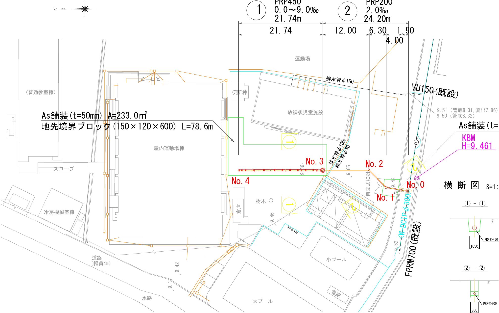
平面図 S=1:500 (大篠小学校)
