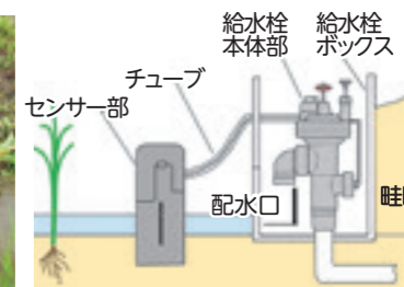
自動給水装置模式図
