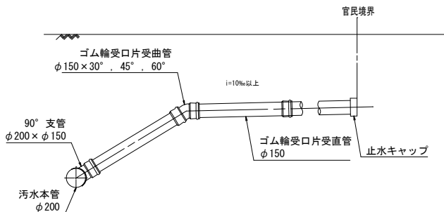
取付管工標準構造図
