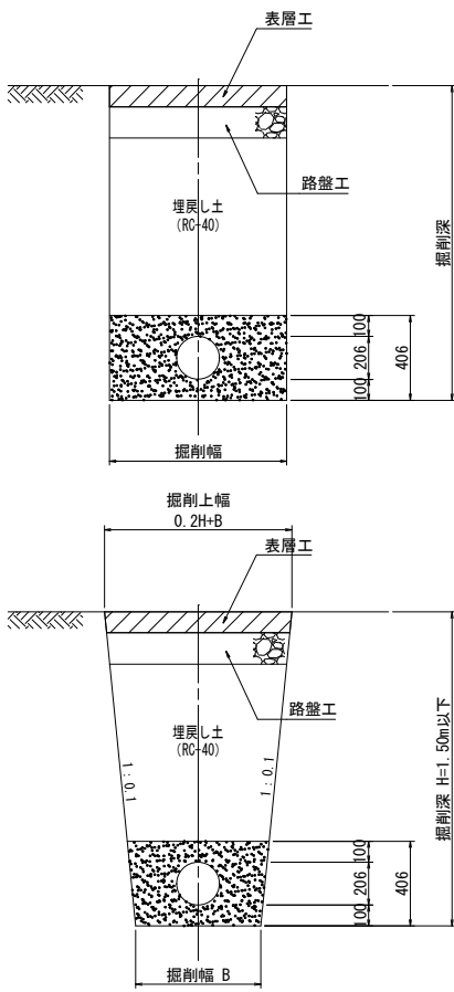
土工定規断面図
