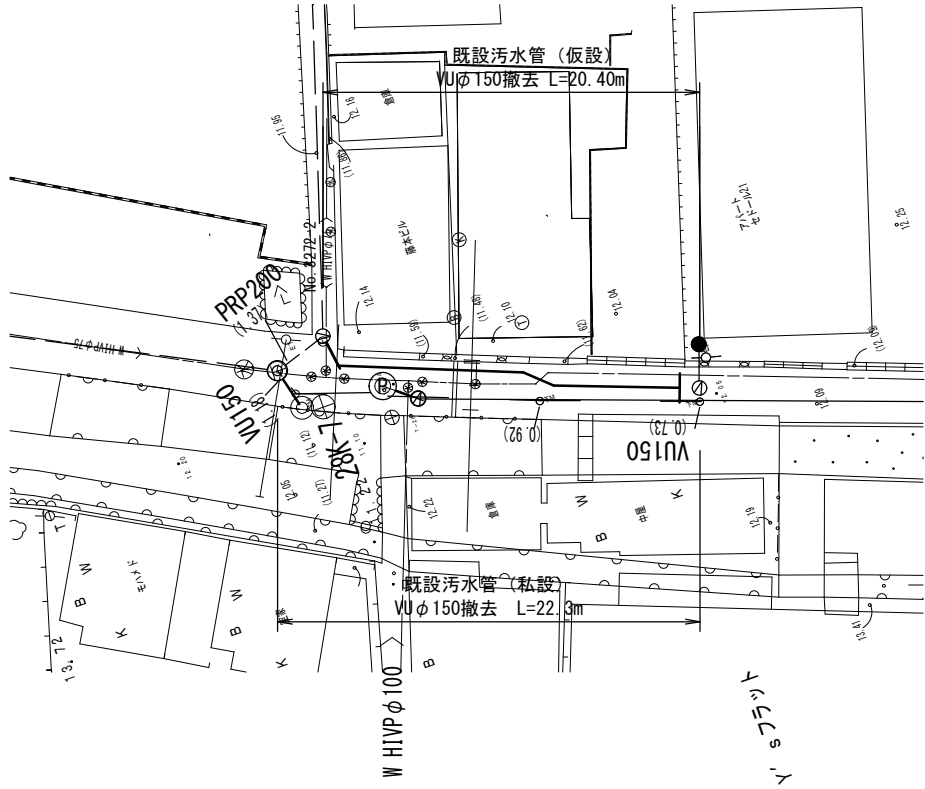
既設管撤去平面図 S=1:200
