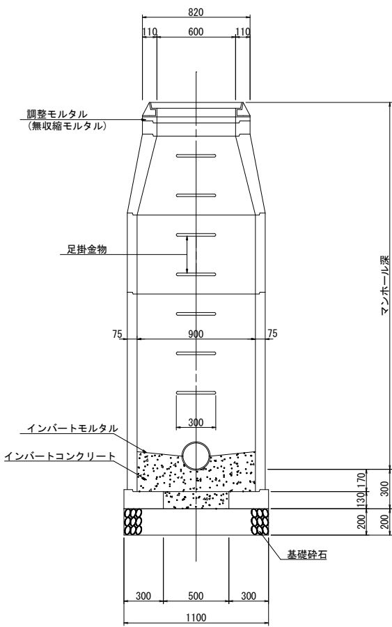
B-B 断面図
