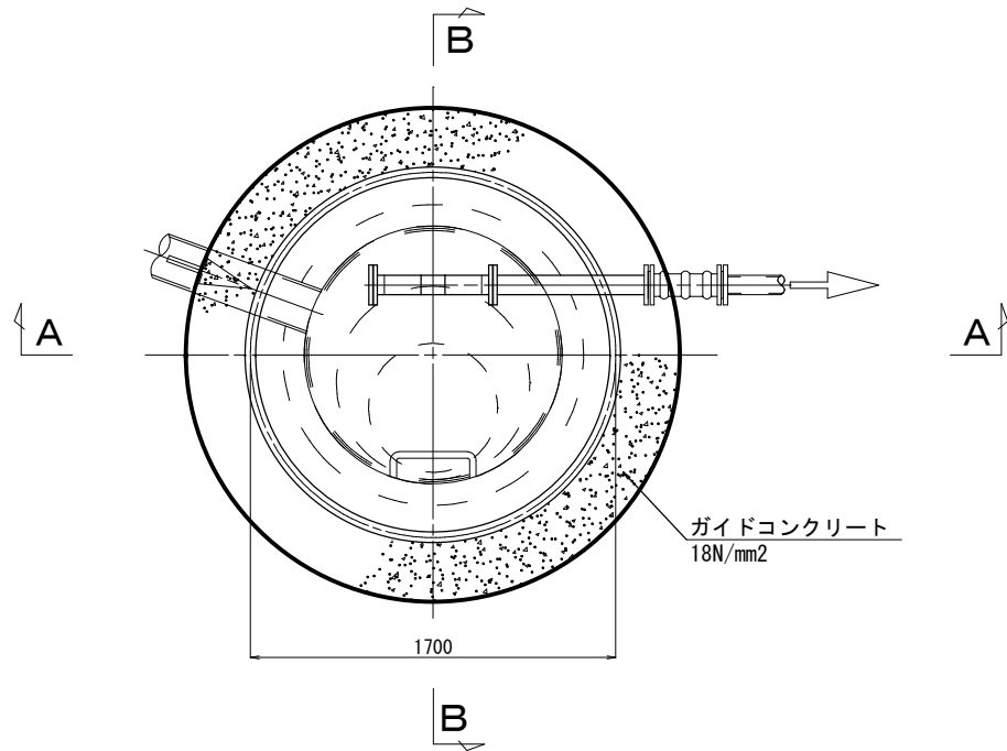
平面图
