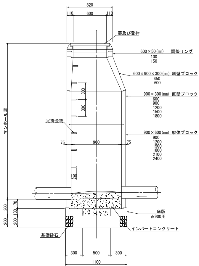
A-A 断面図
