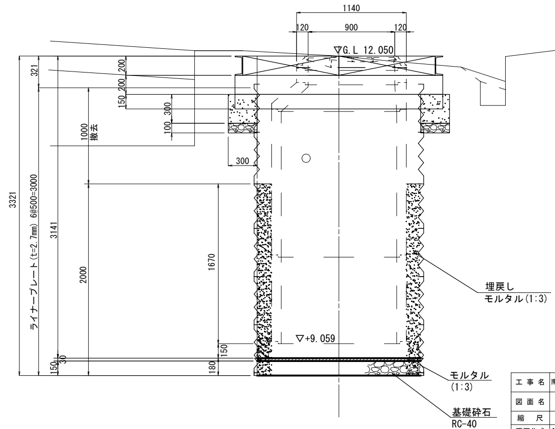
B-B 断面图
